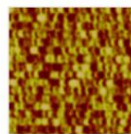
MFM(磁気力顕微鏡)測定結果 (2.5インチ・ハードディスク)
